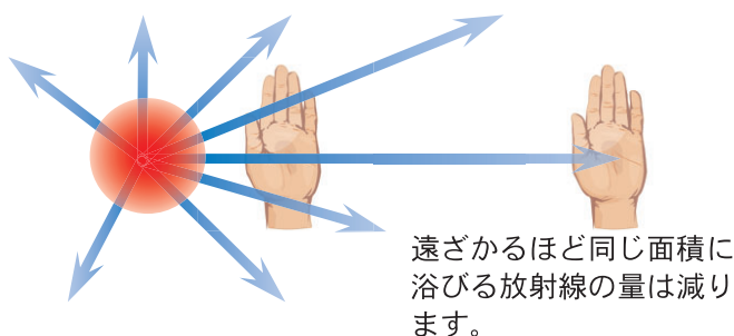
図3 放射線は四方八方に飛びます。
