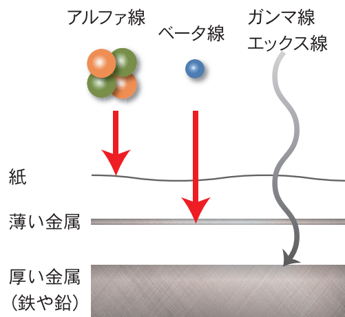
図4 放射線は飛び続けるわけではありません。
